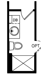
OPTIONAL SHOWER
